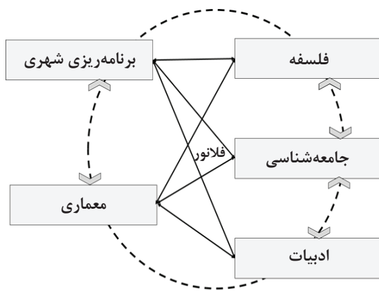
شکل ۱- تقاطع فیلانور و رشته‌های مختلف (منبع: Wang et al., 2024)
