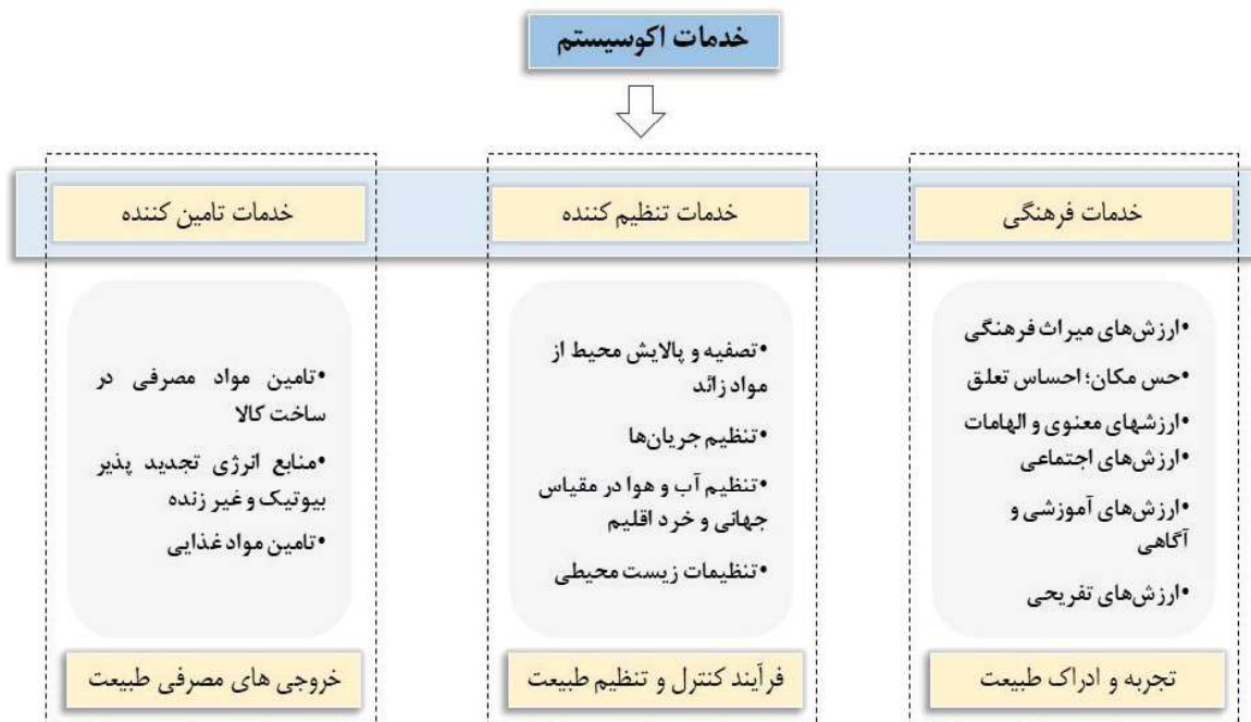
شکل ۲: دسته‌بندی خدمات اکوسیستم (Haines-Young & Potschin, 2011 ،Sukhdev et al., 2010) (Natural England Commis- (Millennium Assessment, 2005 ،sioned, 2011
